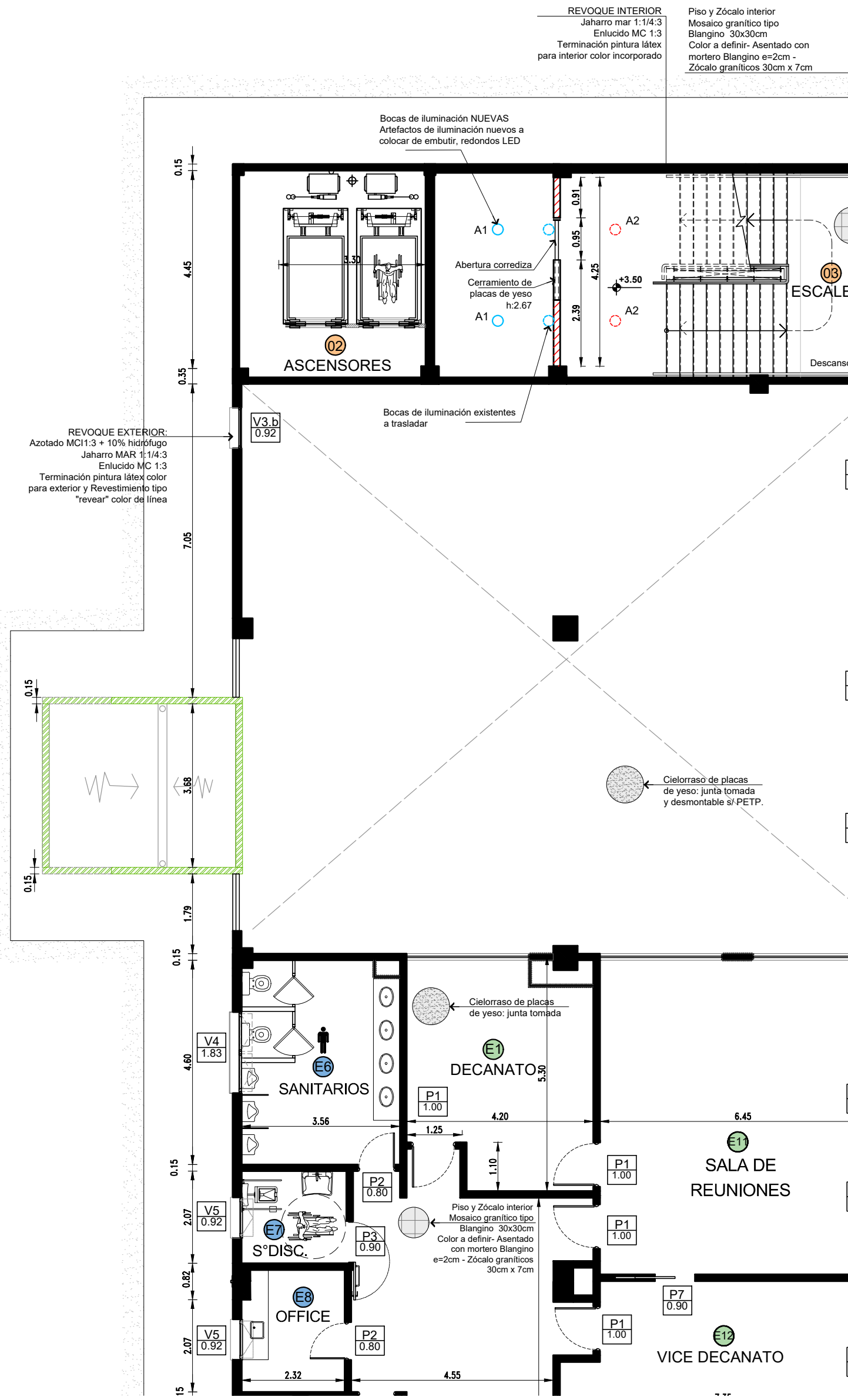
ENTREPISO_PROPOSTA ARCHIVO_ ESC 1:100
