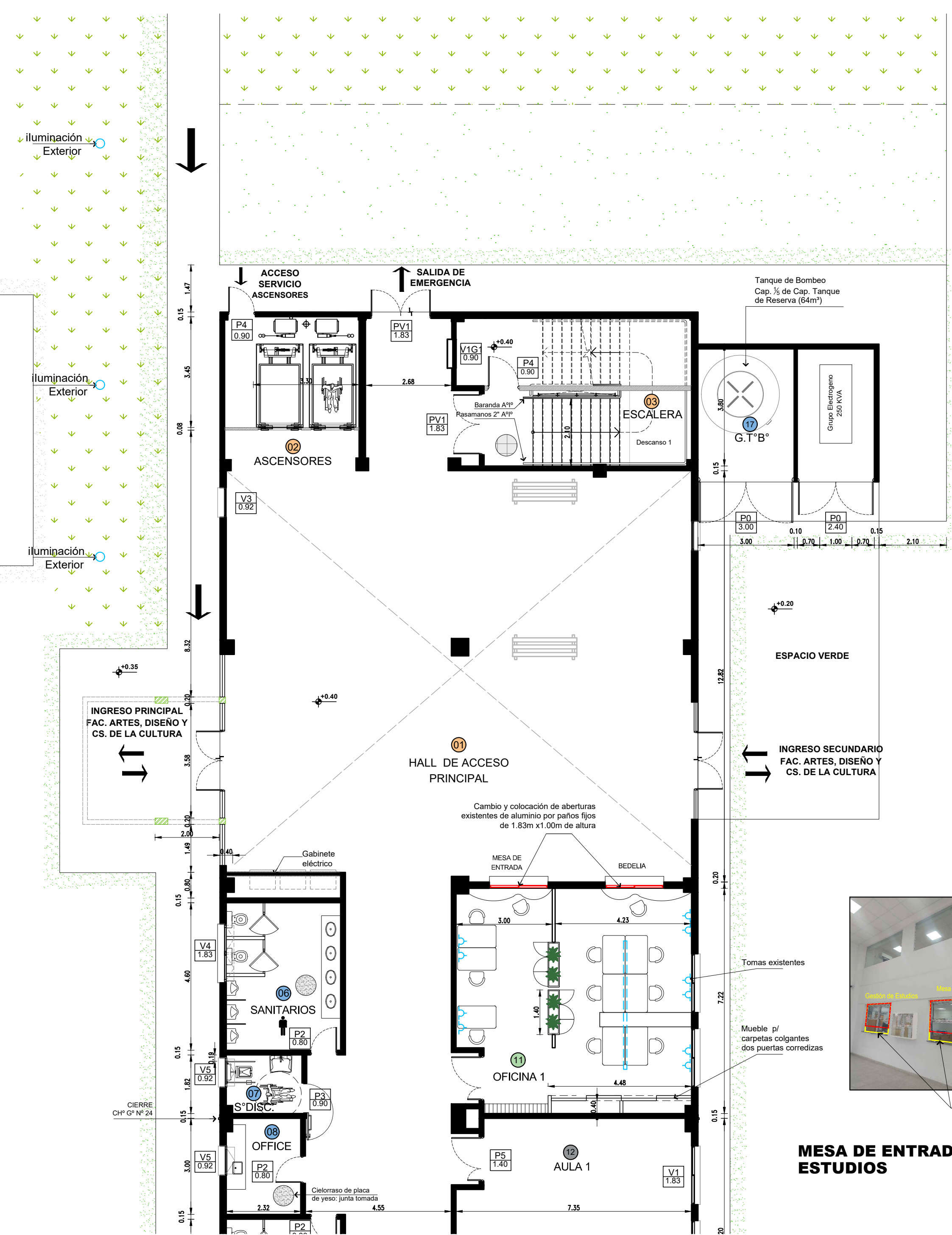
PLANTA BAJA_ Mesa de Entrada y GESTIÓN DE ESTUDIOS ESC 1:100
